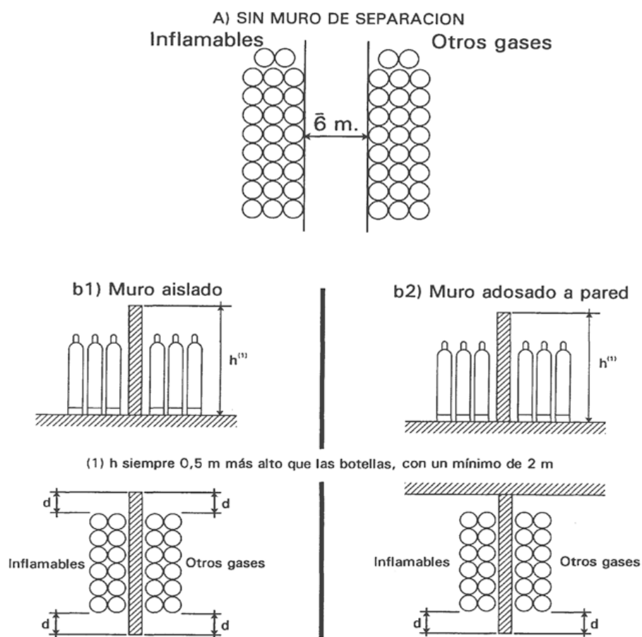
Figura 1: SEPARACION ENTRE BOTELLAS DE GASES INFLAMABLES Y OTROS GASES
